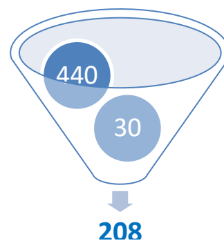
Obrázek 1: Konstrukce slovníku
